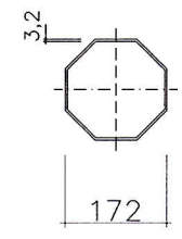
Det. Bottom Of Pole SCALE 1 : 25
