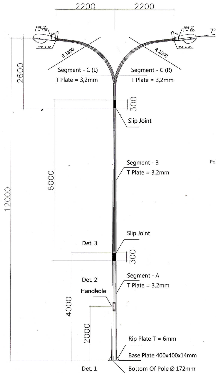
TIANG PJU H-12M DOUBLE PARABOLE SCALE 1 : 25
