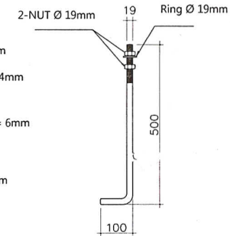
Det. Anchor Bolt SCALE 1 : 25
