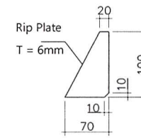
Det. Rip Plate SCALE 1 : 25
