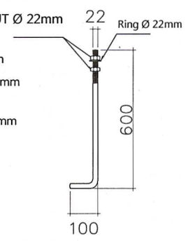
DET 1. ANCHOR BOLT SCALE 1 : 25
