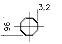
Det. Top Of Pole SCALE 1 : 25
