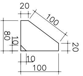
Det. Rip Plate SCALE 1 : 25
