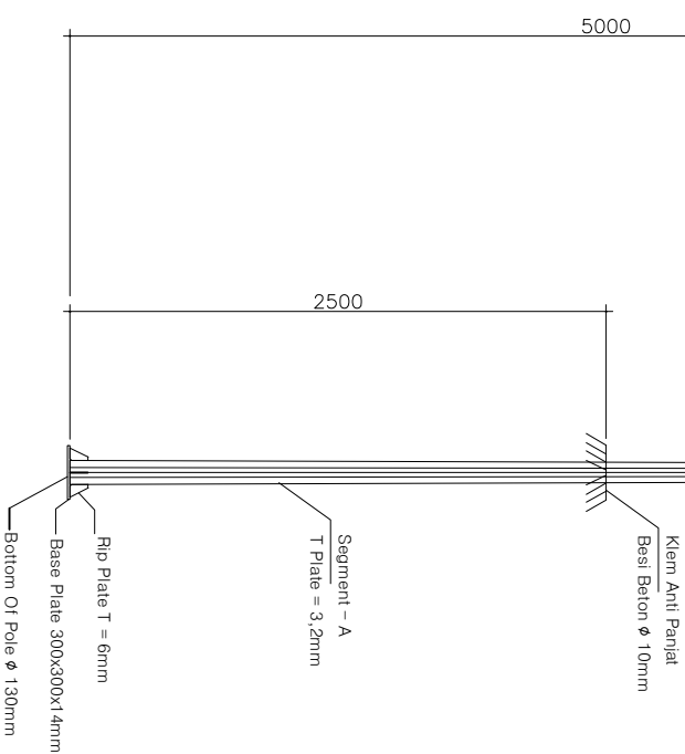
DET 2. Klem Anti Panjait SCALE 1 : 25
